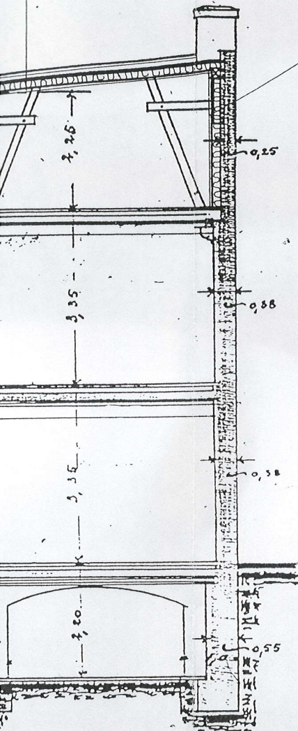
Schnitt a.b.
