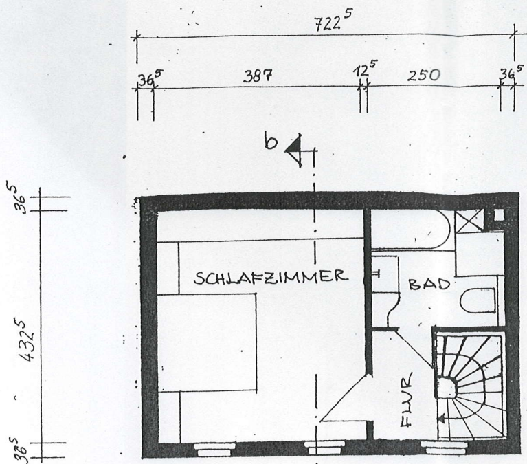
a 2. Obergeschoß
