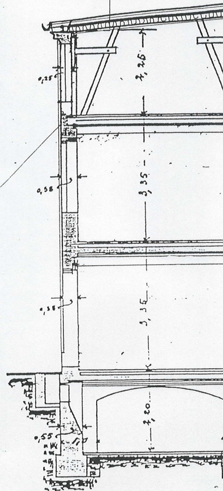
Schnitt a.b.
